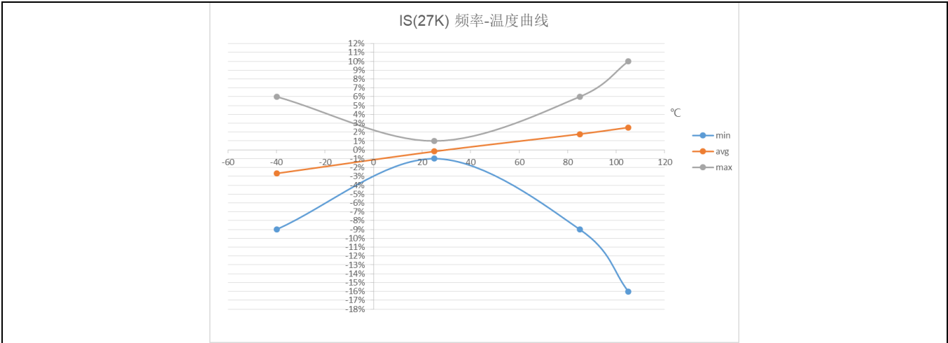
Figure 3-11 IS(27K)频率温度曲线
